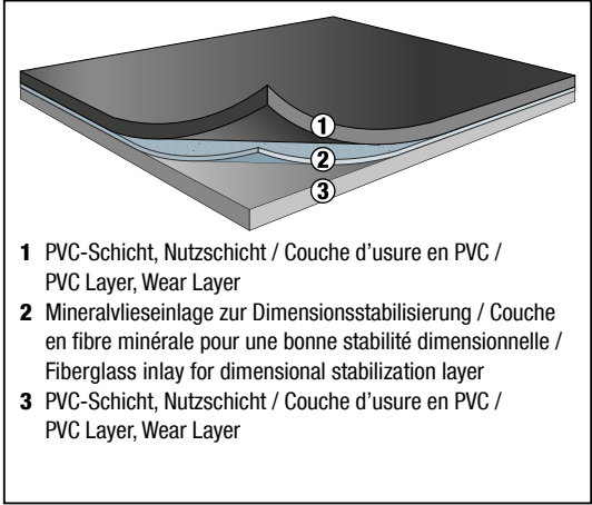
Bodenaufbau / Construction du tapis / Layer Structure
