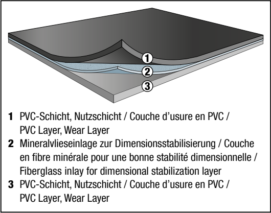
Bodenaufbau / Construction du tapis / Layer Structure
