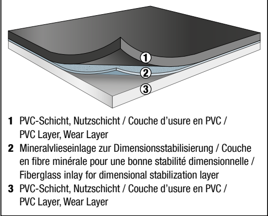
Bodenaufbau / Construction du tapis / Layer Structure
